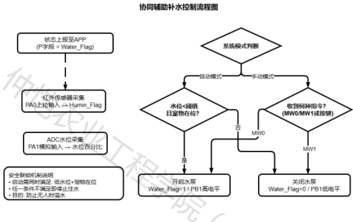
图23 协同辅助补水流程
